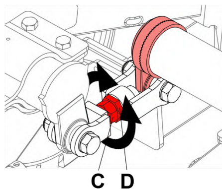
Figure 4.24 – SR460/620 – Réglage grossier et fin des ailes
