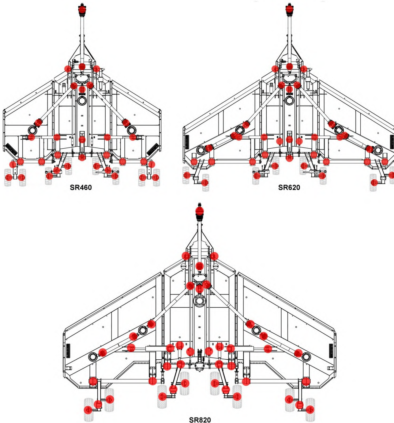
Figure 5.8 – Emplacements des points de graissage
