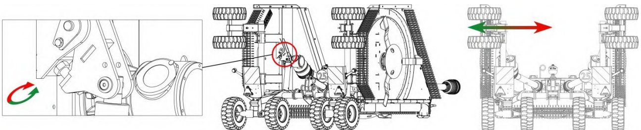
Figure 4.39 – Réglage de la largeur de transport des ailes de la SR460
