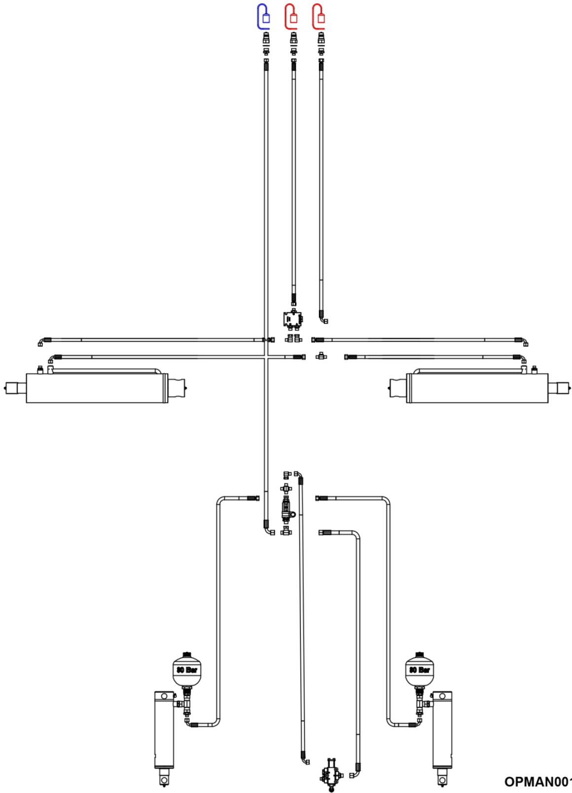
Figure 5.72 – Schéma des flexibles de la SR820
