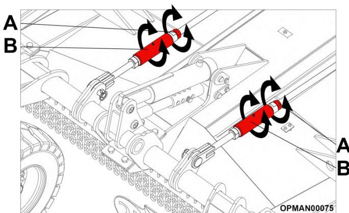
Figure 4.21 – Réglage des barres de liaison (modèle SR460 représenté)
