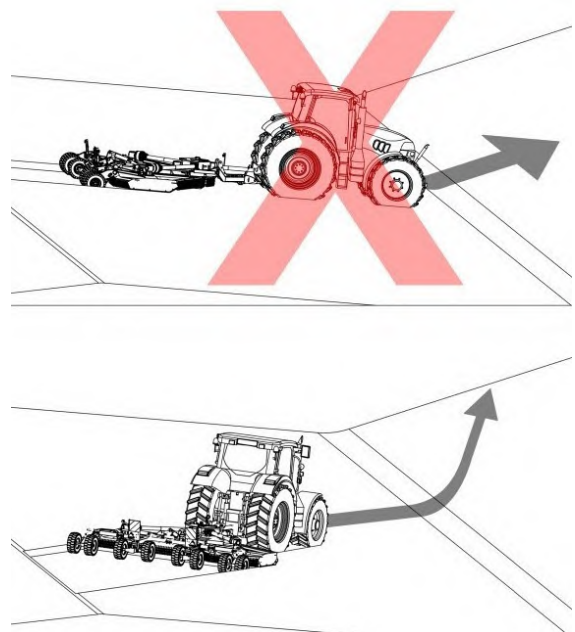
Figure 4.36 – Approcher les fossés obliquement
