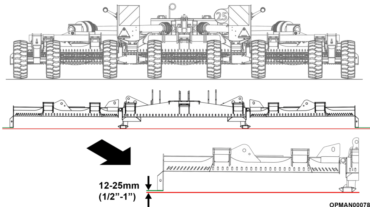
Figure 4.23 – Réglage de hauteur des ailes (modèle SR460 représenté)
