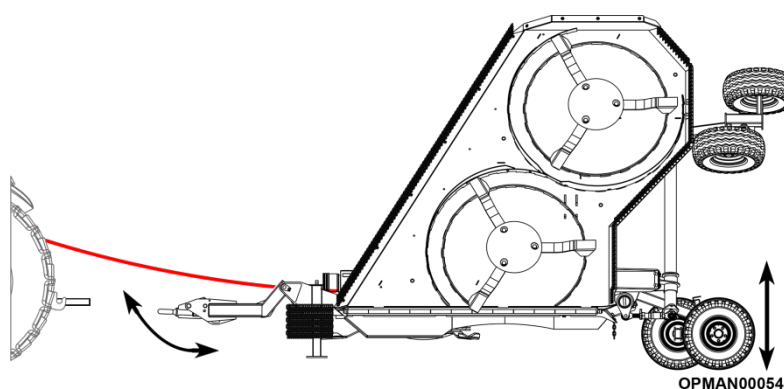
SR820 Figure 4.6 Réglage de hauteur de l'anneau de remorquage
