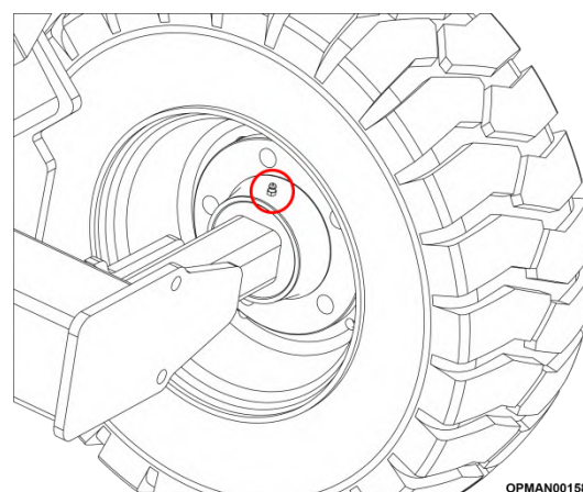
Figure 5.75 – Emplacement de graissage des moyeux de roues SR460/620/820
