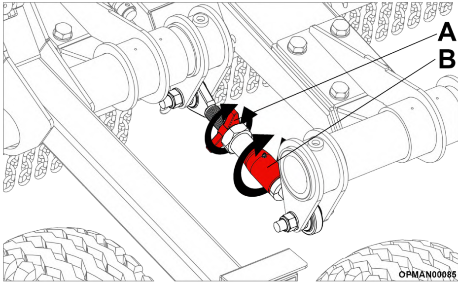
Figure 4.25 – Réglage des ailes de la SR820
