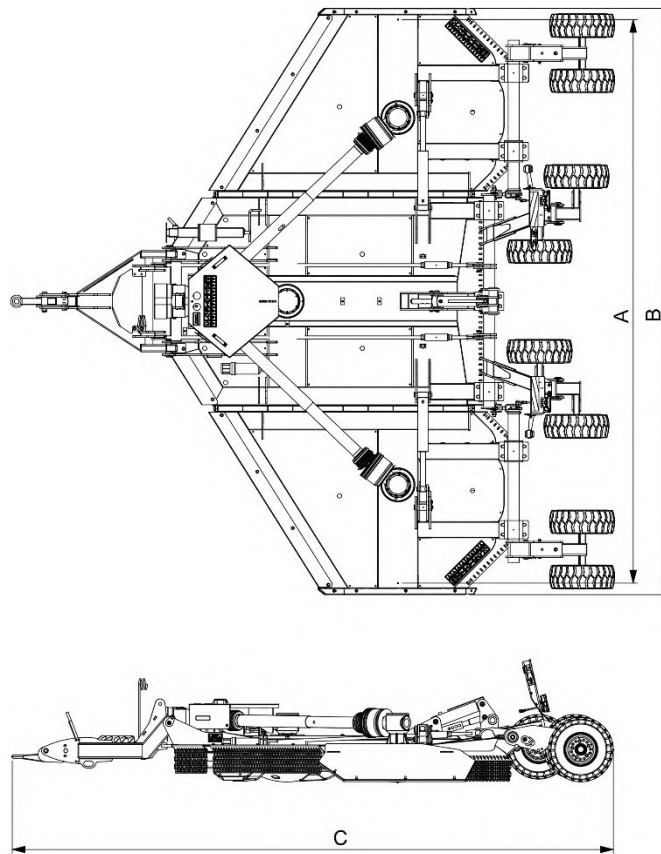
Figure 1.11 Dimensions de travail
