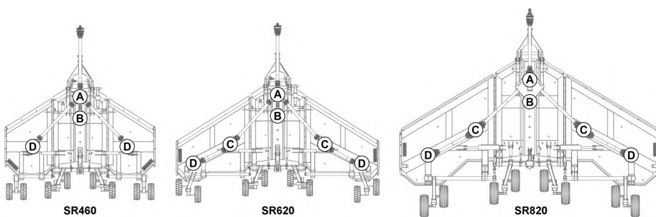
Figure 5.1 – Emplacements de remplissage d'huile des réducteurs des SR460/620/820
