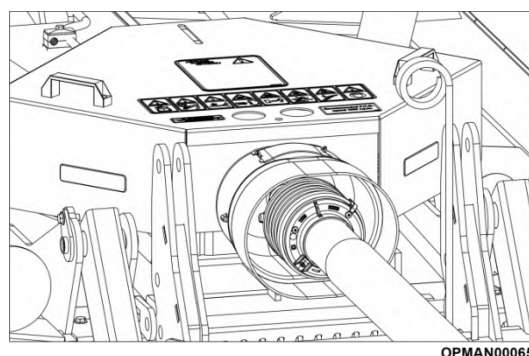
Figure 4.12 – Pose sur Tondeuse
