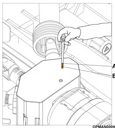
Figure 5.2 – Repères sur la jauge d'huile des SR460/620/820 (il n'est pas nécessaire de déposer la protection)
