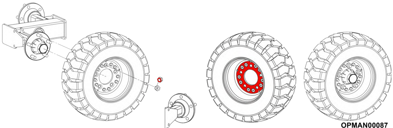
Figure 5.73 – Orientation des roues et des écrous de roues sur les SR460/620/820
