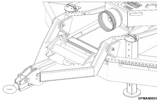
Figure 3.4 – SR820 Positionnement du cric
