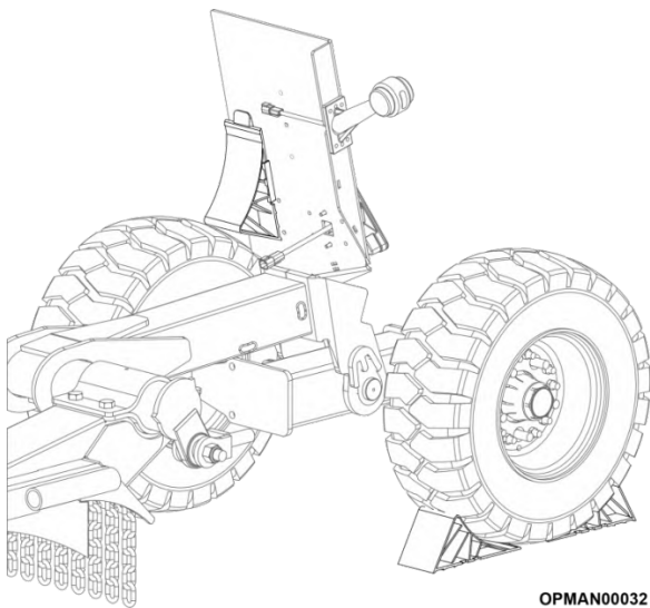
Figure 3.2 – SR460/620 – Rangement et positionnement des cales
