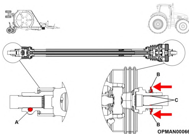
Figure 4.10 – Pose et dépose de l'arbre d'entrée de la SR460/620/820
