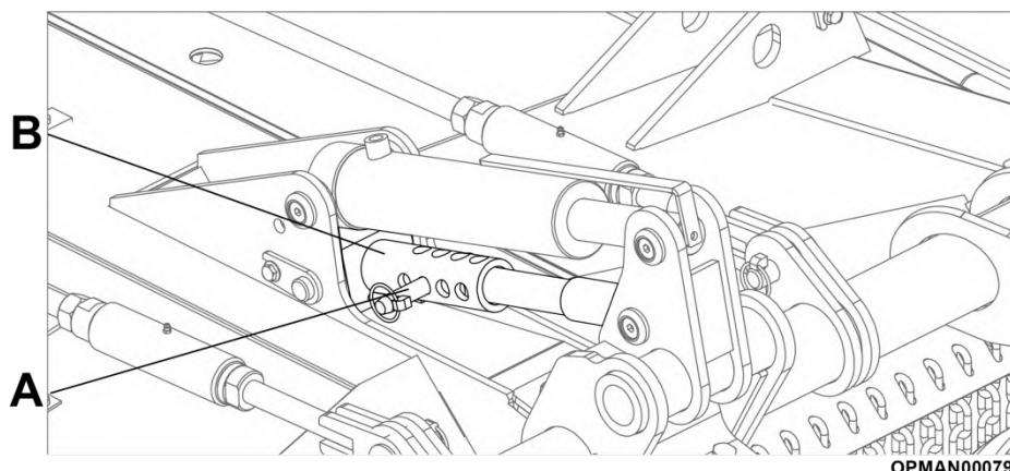
Figure 4.26 – Butée de hauteur minimale de la SR460/620
