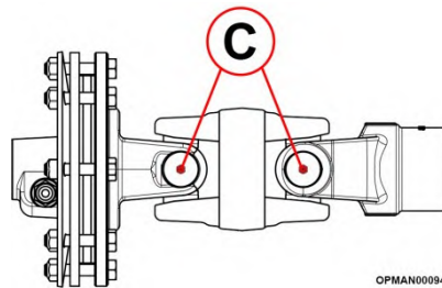
Figure 5.6 – Emplacements des points de graissage d'accouplement central
