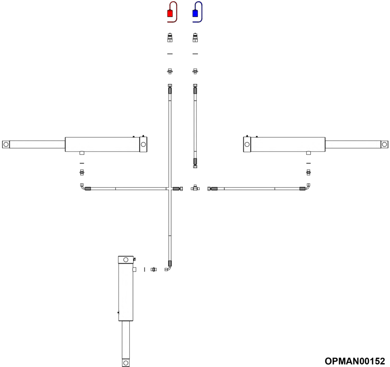
Figure 5.71 – Schéma des flexibles des SR460/620
