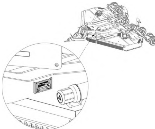
Figure 1.7 – Emplacement de la plaque signalétique (modèle SR460 représenté)
