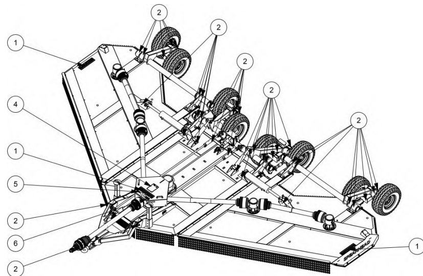
Figure 2.5 – Emplacement des autocollants de sécurité et d'instructions de la SR820
