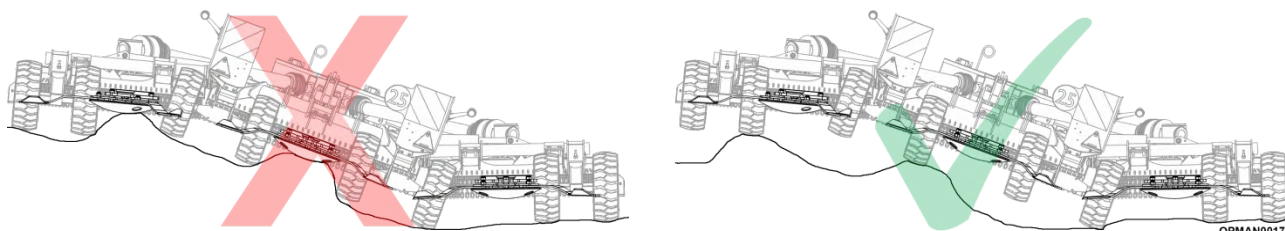
Figure 4.37 – Surface irrégulière, rouler sur les pneus, pas sur le porte-lames
