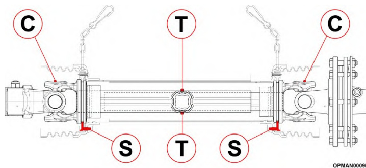
Figure 5.7 – Emplacements des points de graissage d'arbre intérieur/extérieur d'aile
