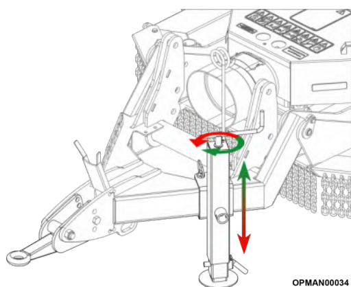
SR460/620 Figure 4.5 Réglage de hauteur de l'anneau de remorquage
