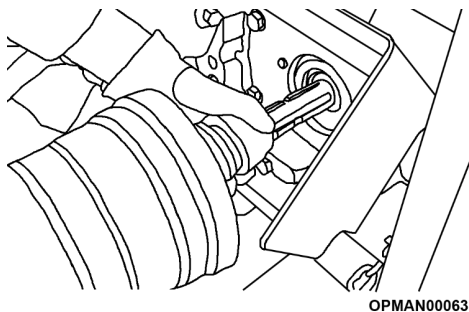
Figure 4.13 – Pose de l'arbre d'entrée sur le tracteur
