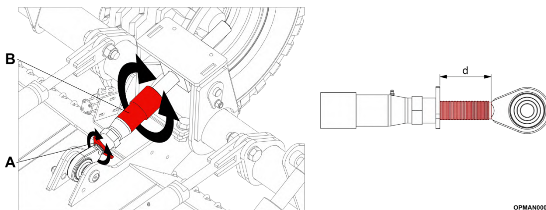
Figure 4.28 – Butée de hauteur minimale de la SR820
