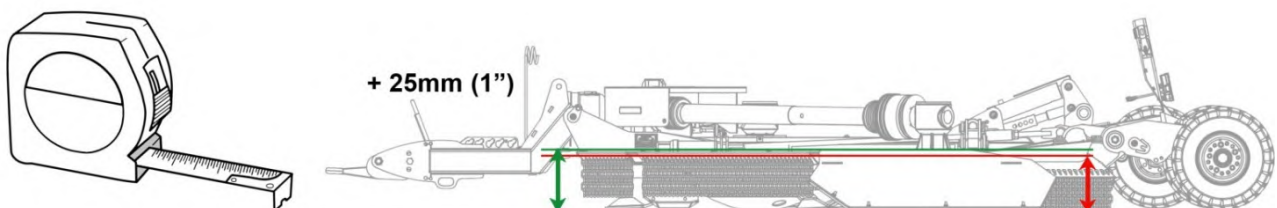
Figure 4.19 – SR460/620 – Mise à niveau avant/arrière de la machine (modèle SR460 représenté)
