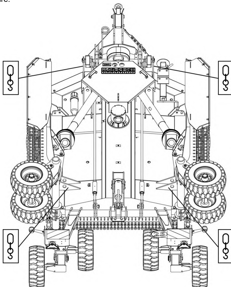
Figure 3.1 Position d'expédition – SR460/620 seulement
