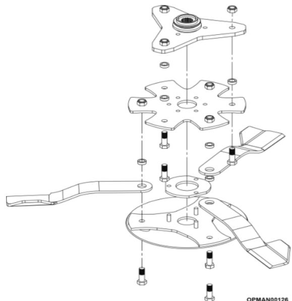
Figure 5.48 – Porte-lames (avec disques Starcut)
