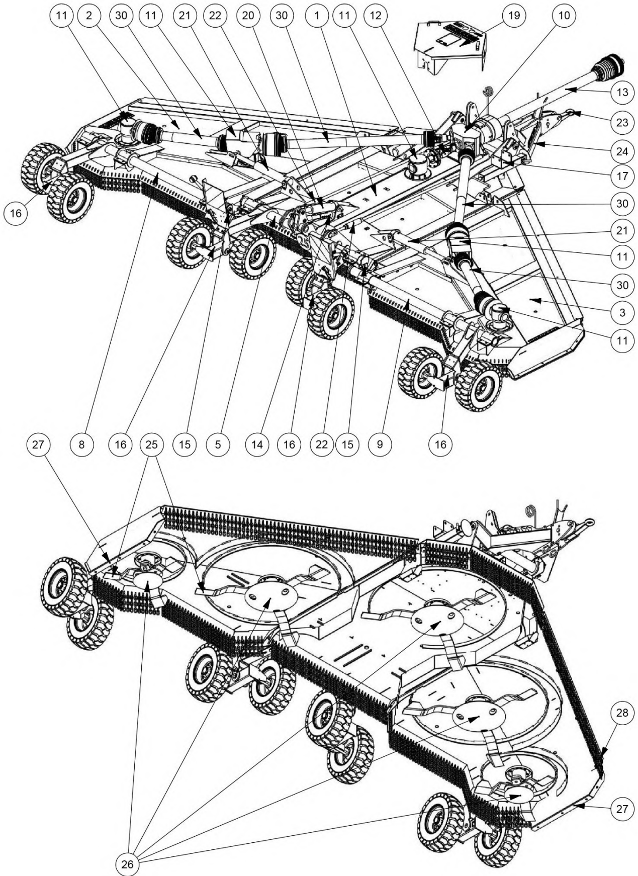
Figure 1.4 – Agencement général de la SR620
