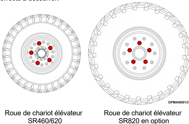
Figure 5.74 – Écrous de roues à desserrer
