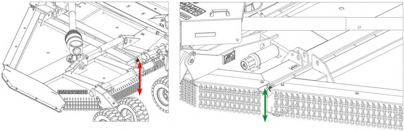
Figure 4.20 – SR460/620 – Mise à niveau avant/arrière de la machine (modèle SR460 représenté)
