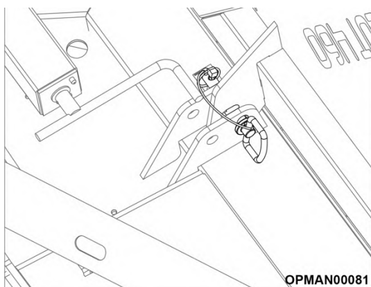
Figure 4.16 SR460/620 – Goupilles de verrouillage des ailes
