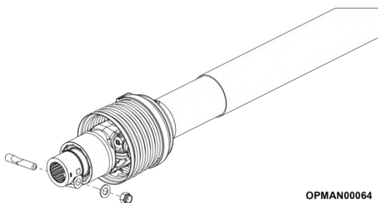
Figure 4.11 – Retrait de la goupille conique
