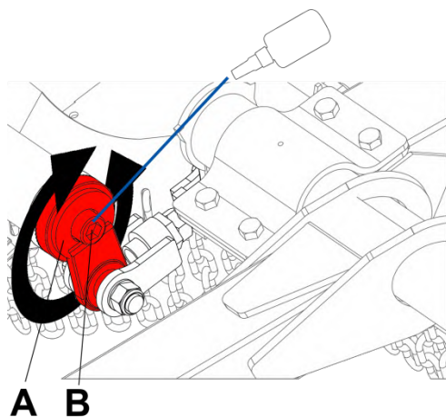
Figure 4.24 – SR460/620 – Réglage grossier et fin des ailes
