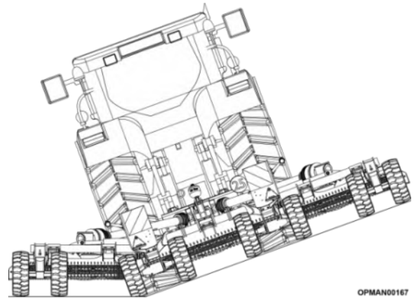
Figure 4.34 – Stabilité du tracteur
