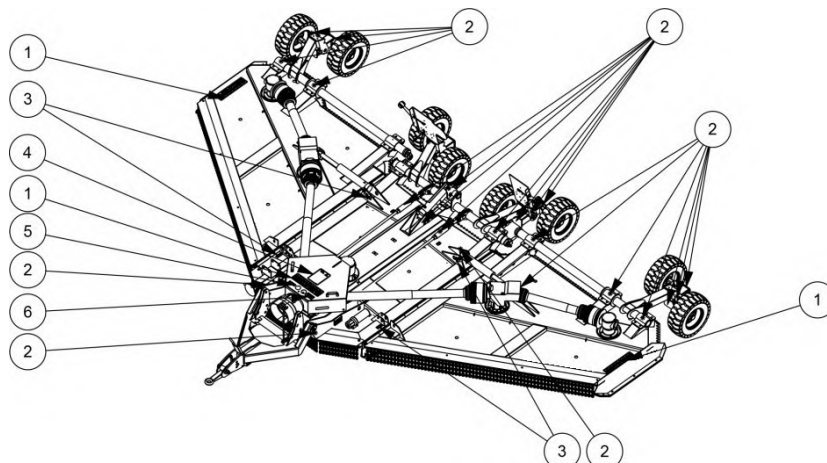
Figure 2.4 – Emplacement des autocollants de sécurité et d'instructions de la SR620
