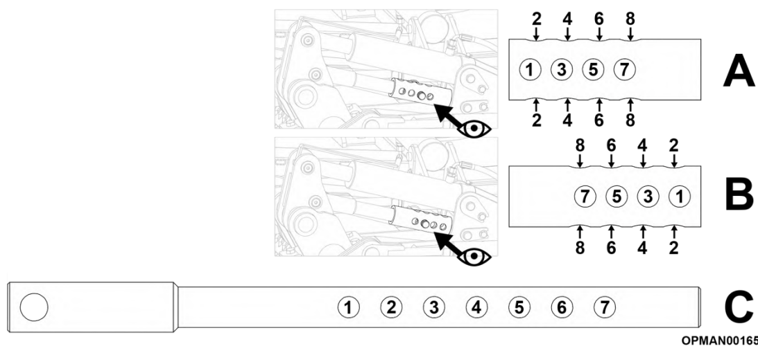
Figure 4.27 – Réglage de la hauteur de coupe des SR460/620
