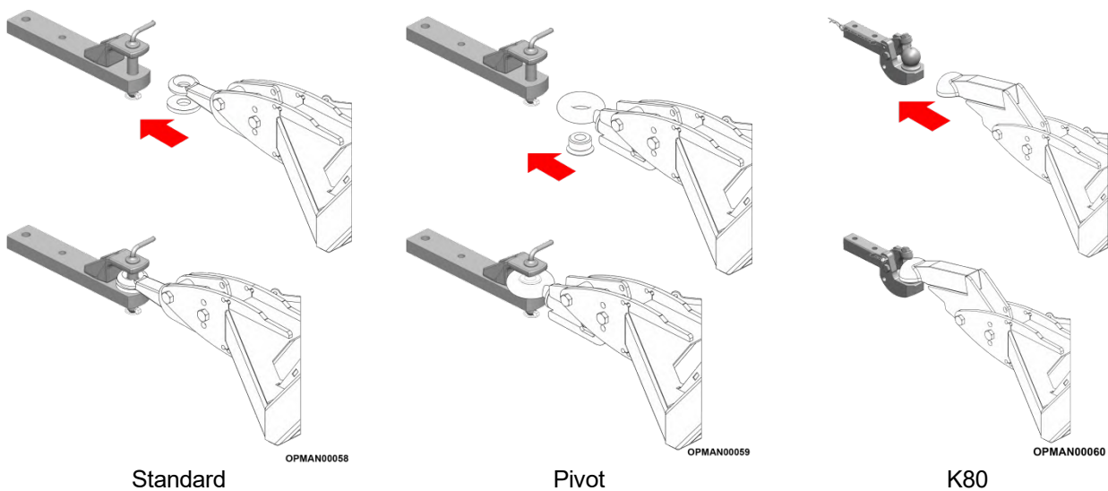
Figure 4.7 – Options d’anneau de remorquage pour SR460/620/820
