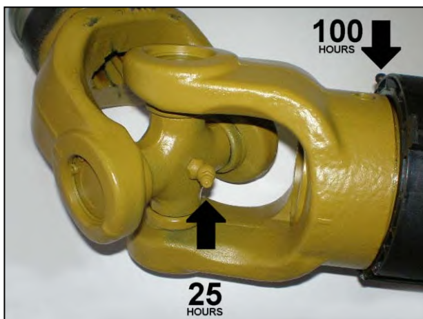
Priporočena pogostost mazanja
