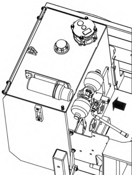
Kit Flottaison placement
