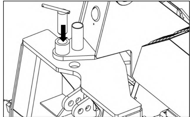
Balayage serrure position – Std. & Tele modèles
