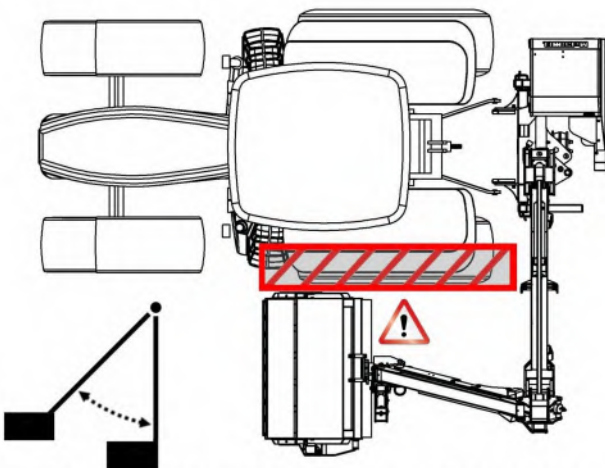
POSITION AVANT - ZONE DE RISQUE DE CONTACT
