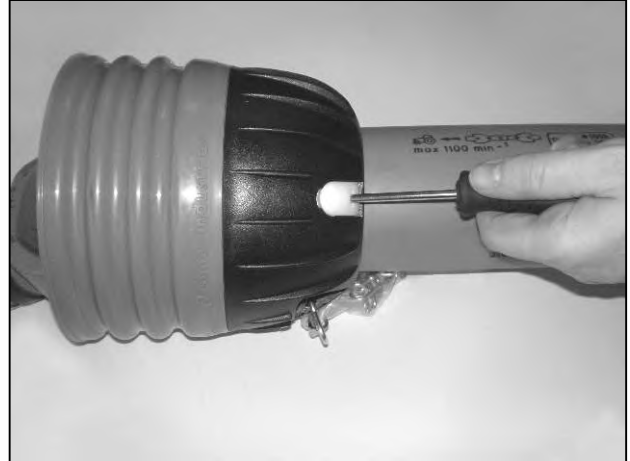
Insérez les tournevis dans les fermeurs
