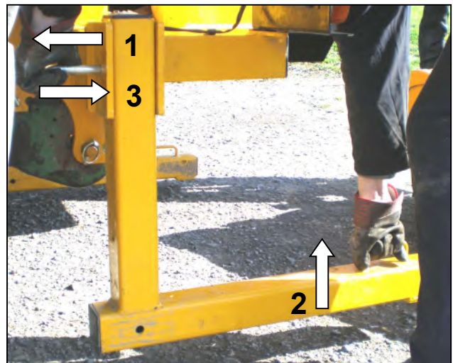
Verwijder steunpoten aan beide zijden van de machine.
